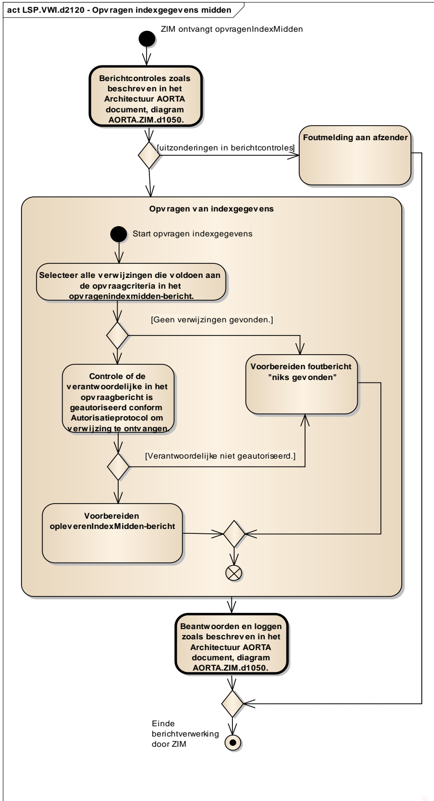
Diagram LSP.VWI.d2120 - inhoudelijke afhandeling service opvragen index midden
