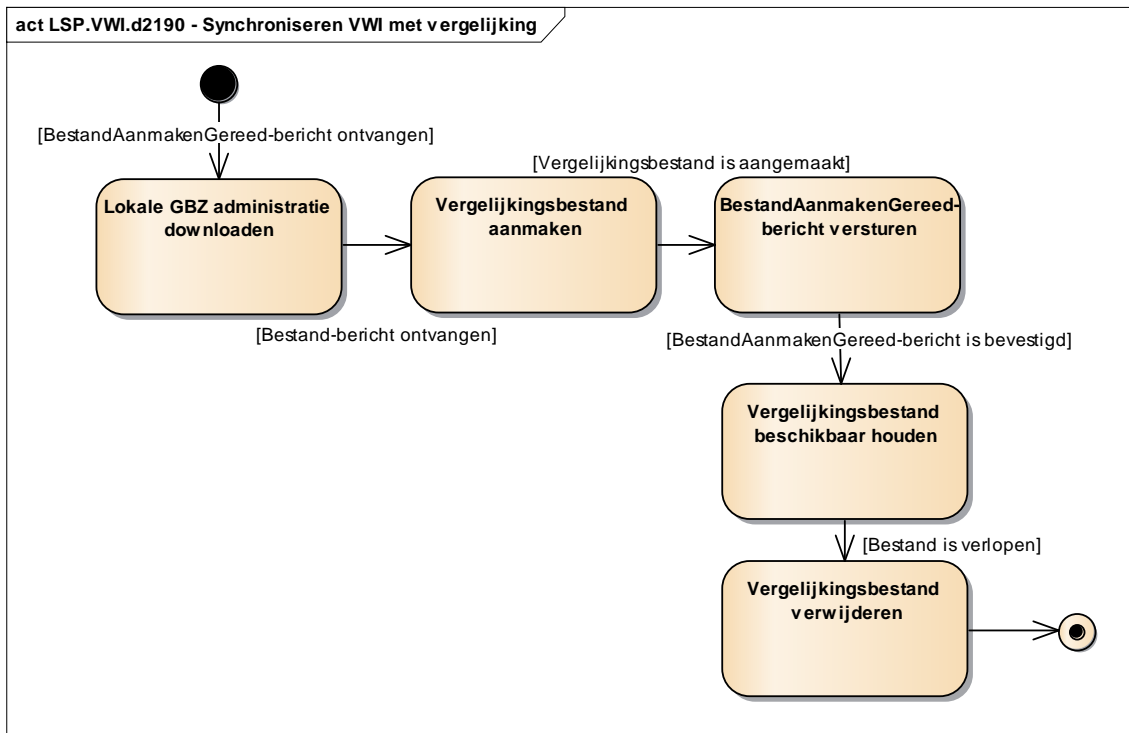
Diagram LSP.VWI.d2190: Synchroniseren VWI met vergelijking
