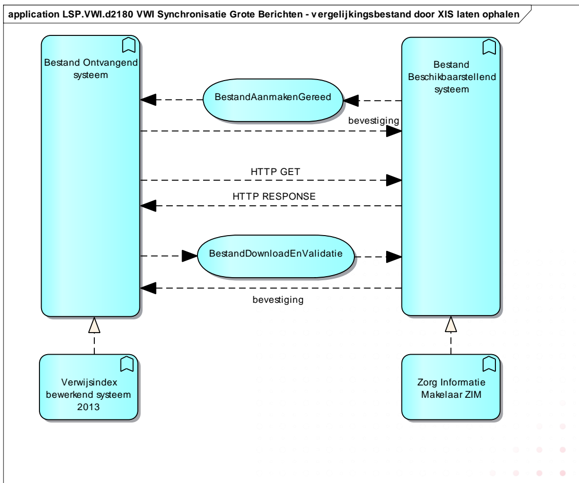
Diagram LSP.VWI.d2180 – Afhandelen van interface Synchroniseren indexgegevens – vergelijkingsbestand door XIS laten ophalen
