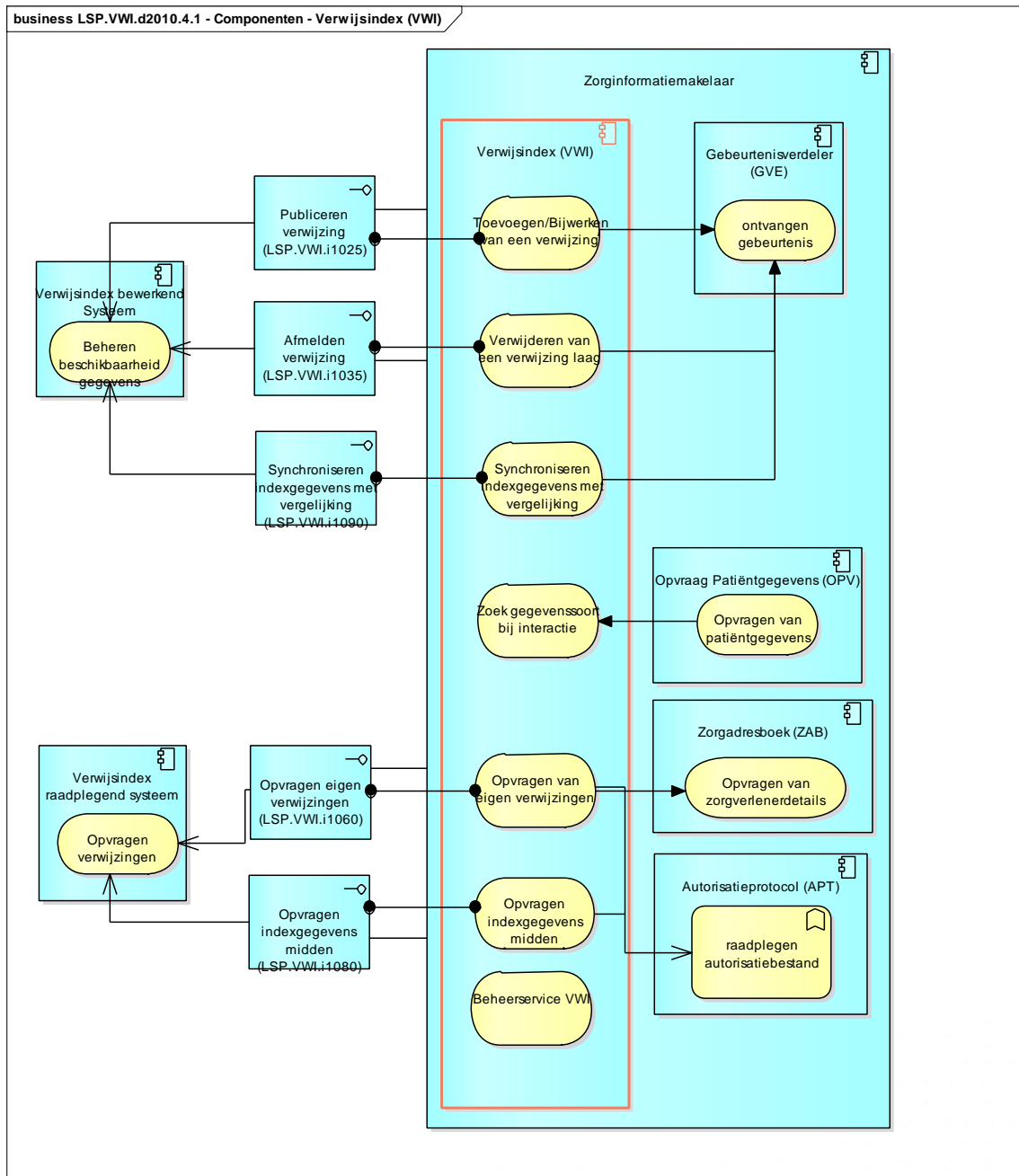
Diagram LSP.VWI.d2010 - interacties met de ZIM
