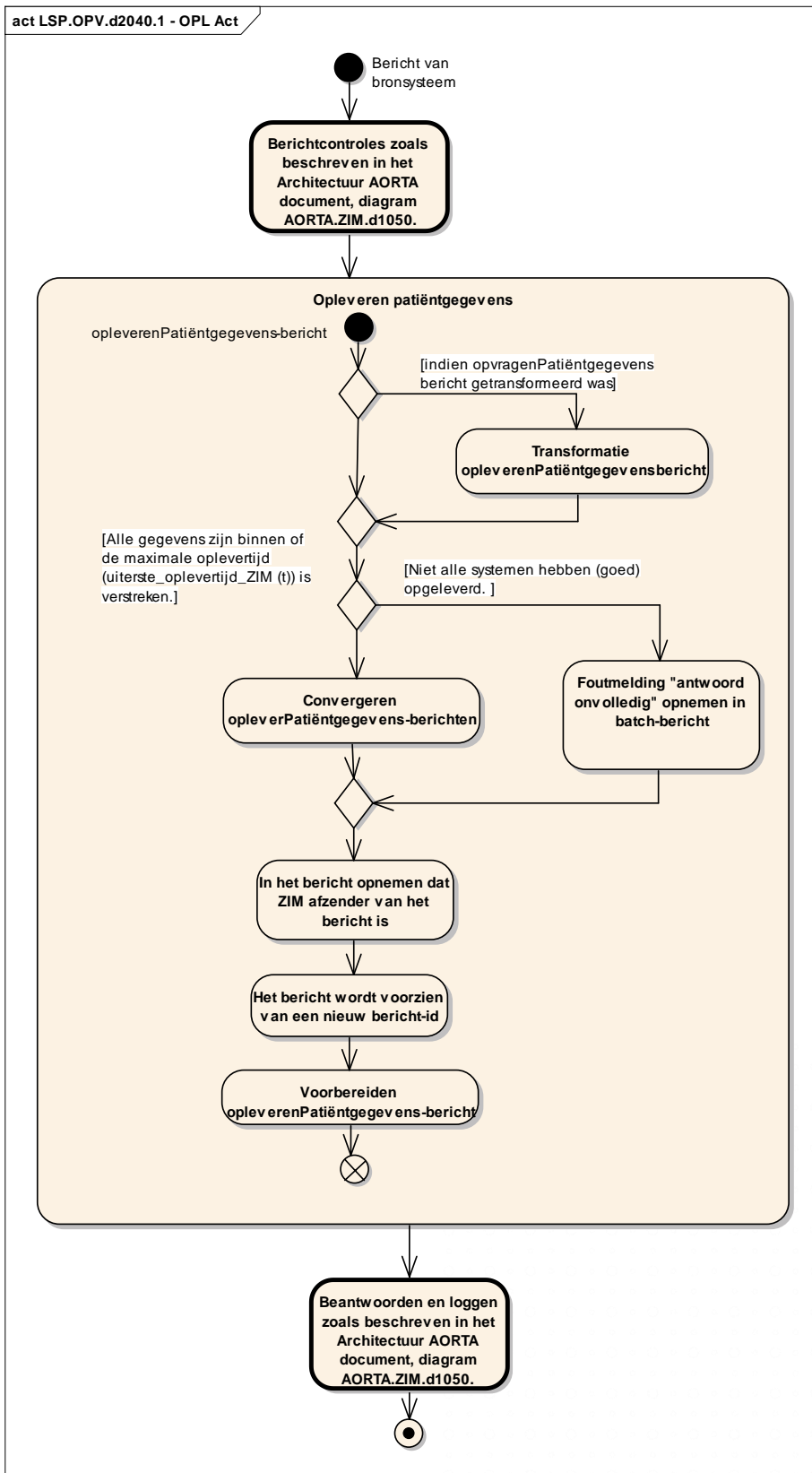
Diagram LSP.OPV.d2040 : Afhandeling opleveren patiëntgegevens in ZIM
