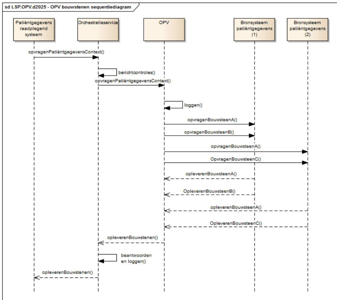
Diagram LSP.OPV.d2025 – OPV context sequentiediagram
