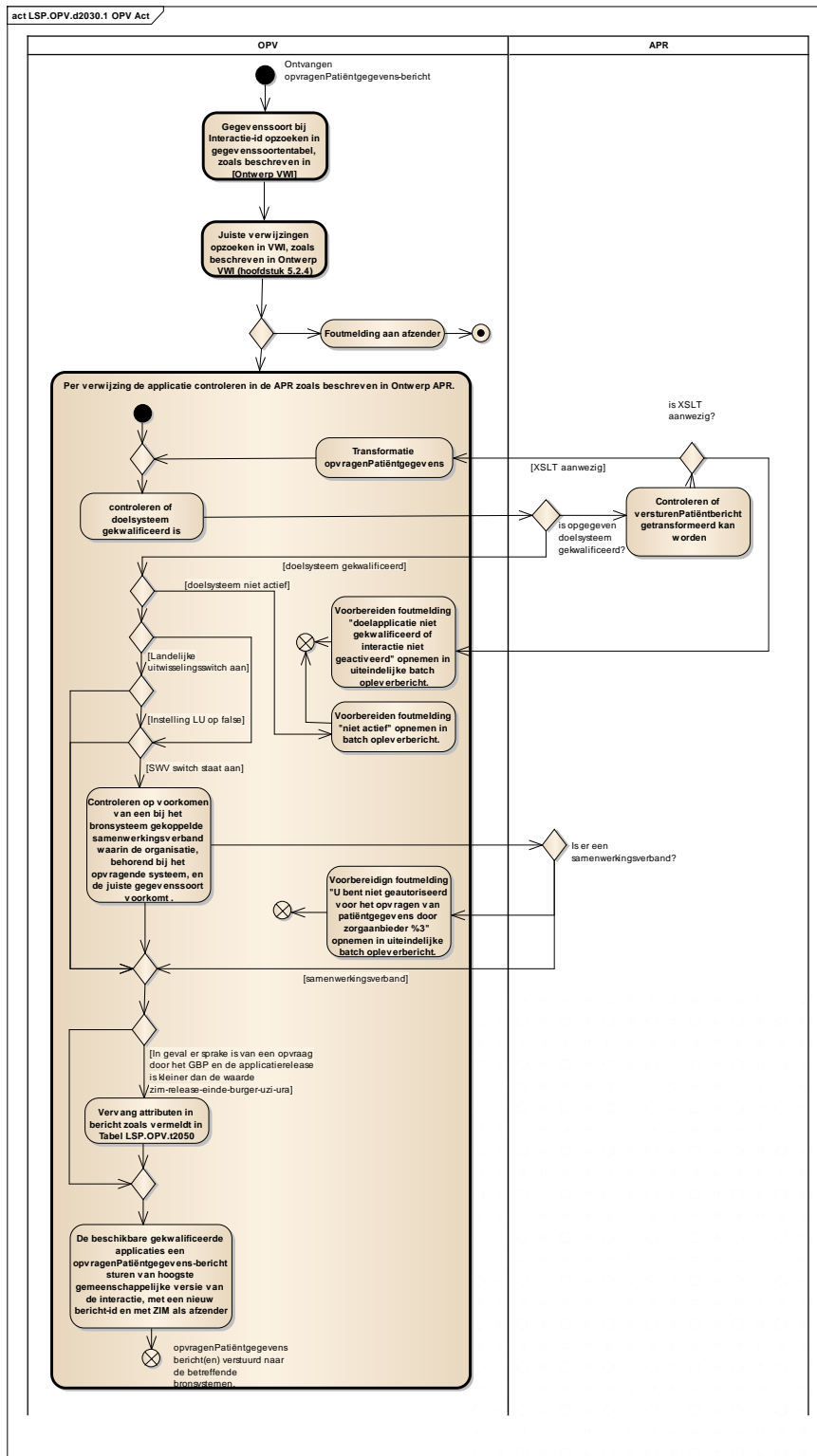
Diagram LSP.OPV.d2030.1 - Opvragen van patiëntgegevens.
