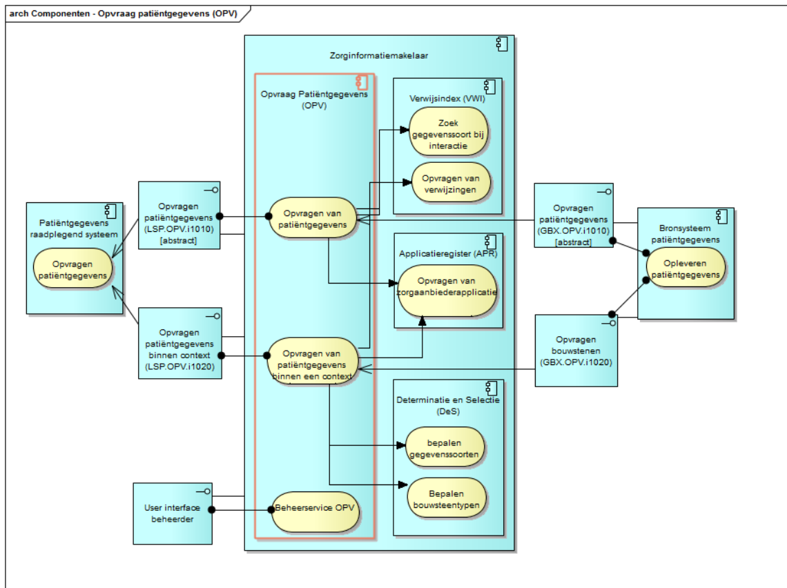
Diagram LSP.OPV.d2010 – interacties met de ZIM
