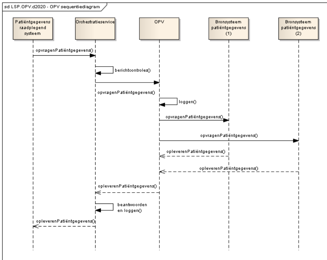
Diagram LSP.OPV.d2020 – OPV sequentiediagram
